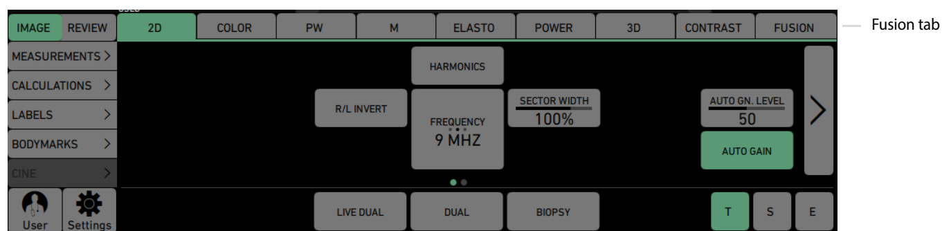
Figure 2-7. Fusion tab
